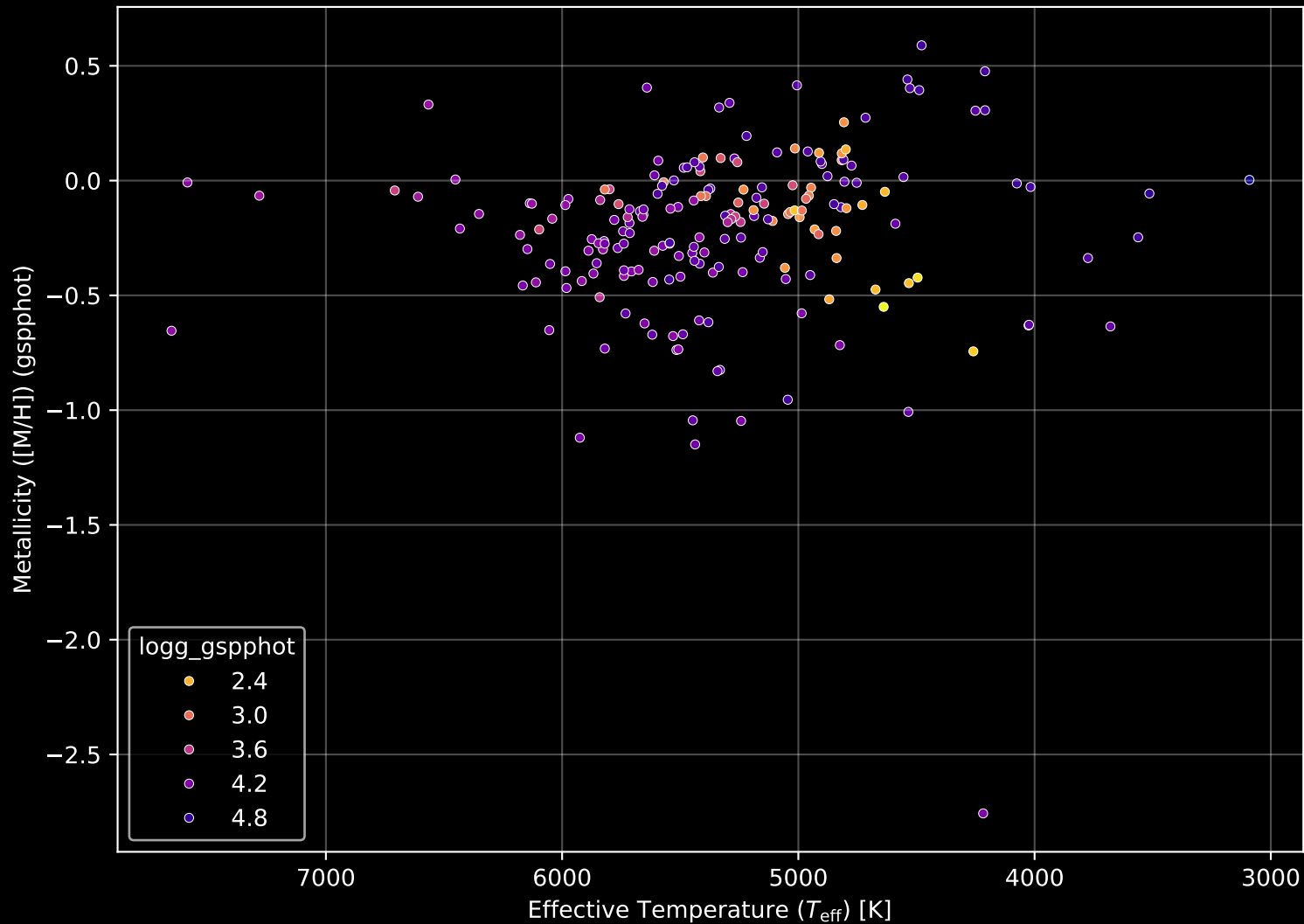
APOGEE DR17 Field: [087-41_MGA] Stellar Population Parameters (n= 198)
